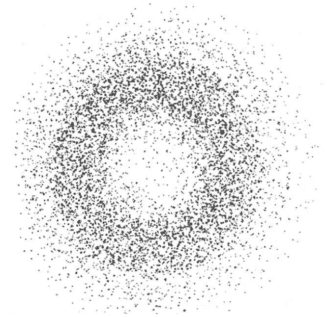
Sekil 11 Bir hidrojen atomunun en düşük yörüngesindeki konumunun tekrarlanan ölçümlerinin sonuçları. Elektron dalgasının sıklıkla onu bulma olasılığının yüksek olarak tahmin edildiği yerde çöktüğü açıktır, böylece kırçıl (bulanık) bir yörünge ortaya çıkar.
